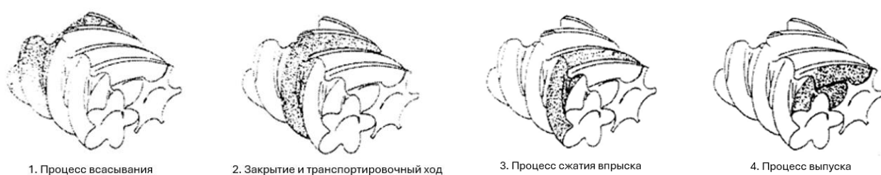
Рис. 1 Принцип сжатия
